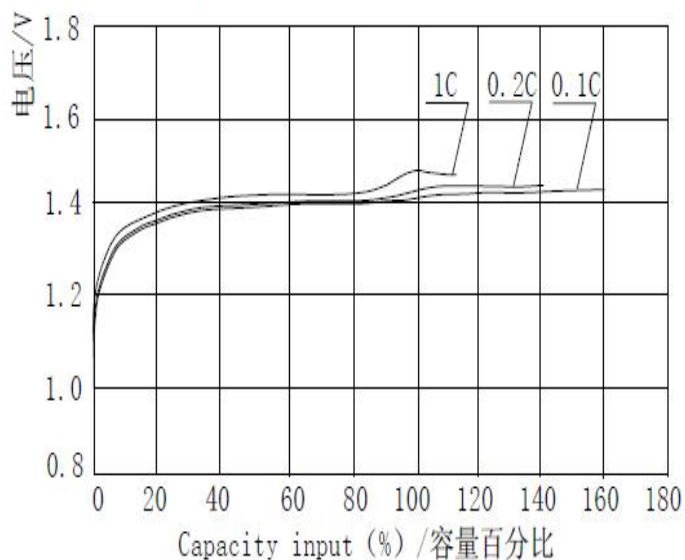
Low rate discharge/低倍率放电
