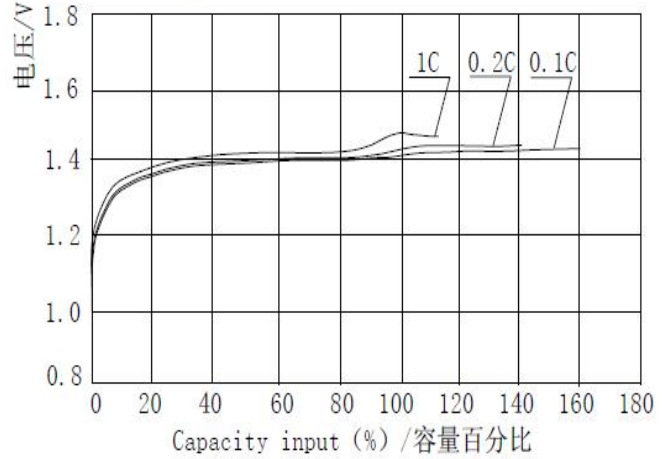
Charge curve/充电曲线
