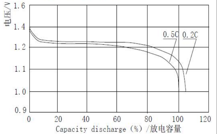
Low rate discharge/低倍率放电
