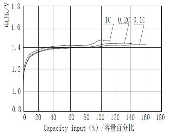
Charge curve/充电曲线
