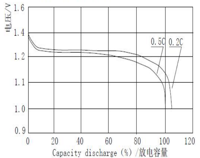
Low rate discharge/低倍率放电
