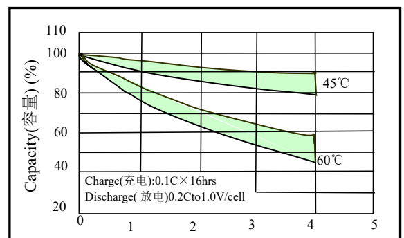
Storage & self discharge Curves 不同温度荷电保持曲线图
